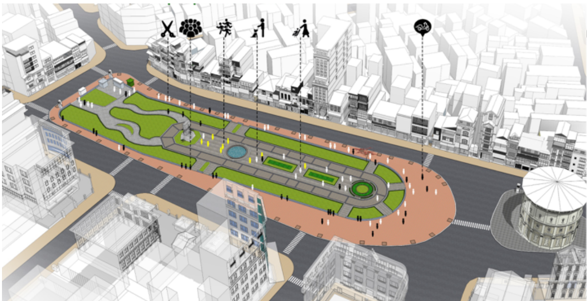
Hình 3.16. Mặt bằng tổng thể vườn hoa Vạn Xuân
